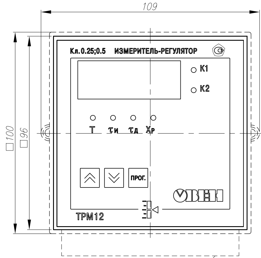
Вид спереди
