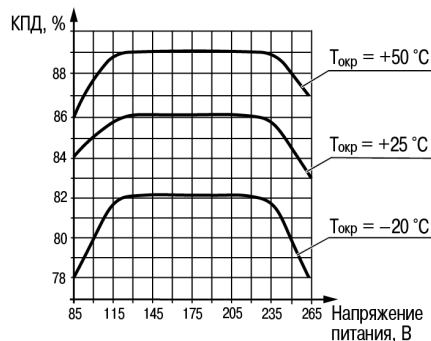
Рисунок 7 - График зависимости КПД от напряжения питания и температуры окружающей среды: (1) БП30А-12, (2) БП30А-24
