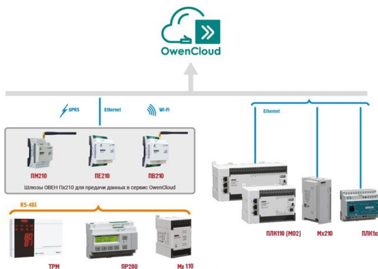
Рисунок 2.2 – Структурная схема подключения устройств пользователя к OwenCloud
