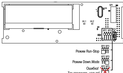
Рисунок 5 – Вид на верхнюю плату со снятой крышкой
