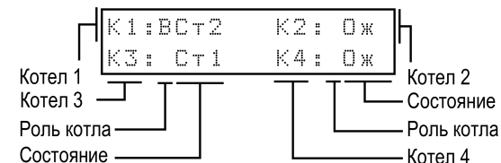
Рисунок 9.8 – Отображение ролей котлов на индикаторе
