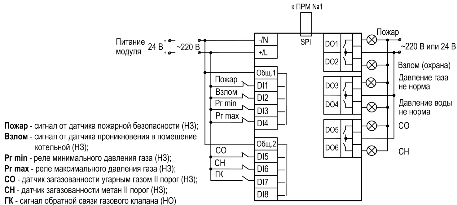
Рисунок 6.6 – Схема подключения к ПРМ-1 сигналов общекотельных аварий
