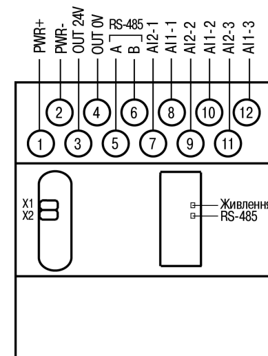
Рисунок 1 – Назначение контактов клеммника
