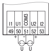
Рисунок 7 – Підключення активного датчика з виходом типу «Напруга 0...10 В»
