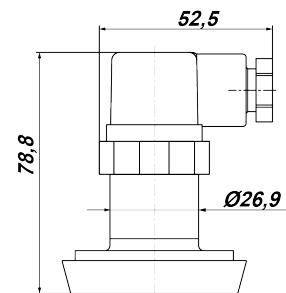
Рисунок 1 – Габаритные и присоединительные размеры ПД180-ДИ, -ДВ, -ДИВ с присоединением Clamp DIN 32676
