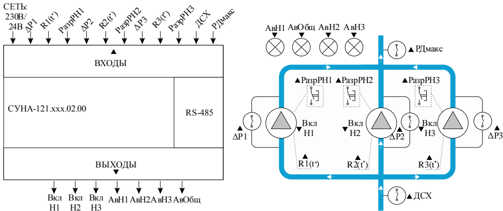
Рисунок 2.1 – Схема объекта управления
