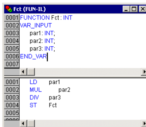
Рисунок 4.2 – Пример записи функции на языке IL
