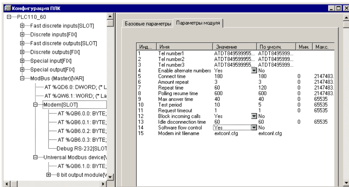
Рисунок Д.2 – Параметры подмодуля «Modem» в режиме «дозвона»
