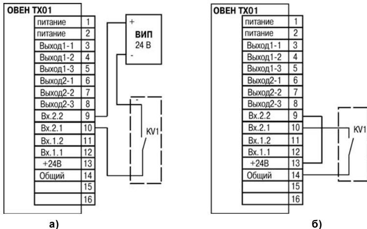
Рисунок Б.1 – Подключение к входу коммутационных устройств:
