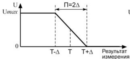
а) обратно-пропорциональное регулирование
