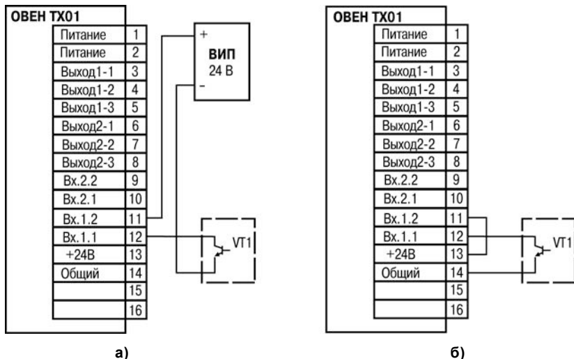
Рисунок Б.2 – Подключение пассивных датчиков, имеющих на выходе транзистор n-p-n типа с открытым коллекторным входом: а) при работе датчика от внешнего источника питания; б) при работе датчика от питающего напряжения прибора
