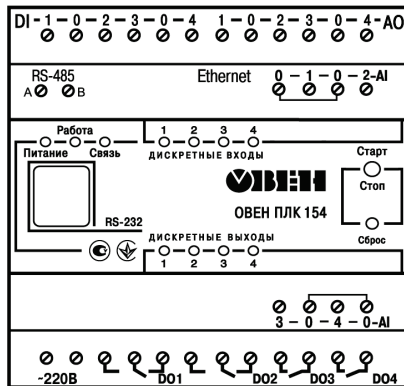
Рисунок 4.1 – Внешний вид контроллера
