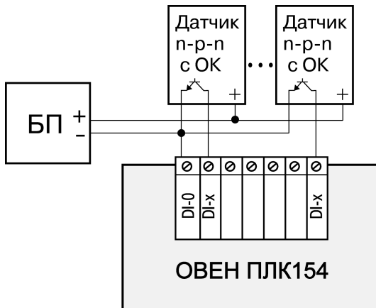
Рисунок Б.2 – Схема подключения к ОВЕН ПЛК154 дискретных датчиков с полупроводниковым выходным каскадом
