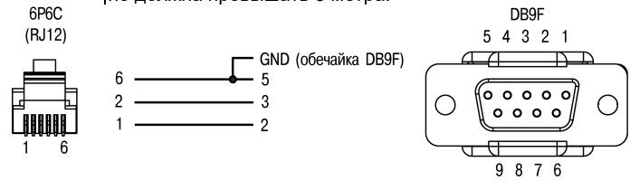
Рисунок В.4 – Кабель KC2 для подключения ОВЕН ПЛК154 к панелям ИП320, СП270 и СП3хх (порт RS-232 Debug)
