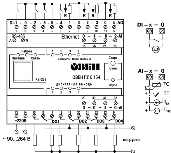
Рисунок Б.1 – Схема подключения питания, входов и выходов к ОВЕН ПЛК154-220.X-X
