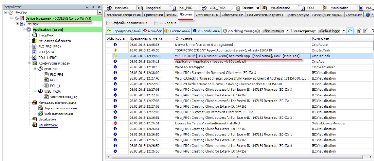
Рисунок 8.17 – Журнал контроллера
