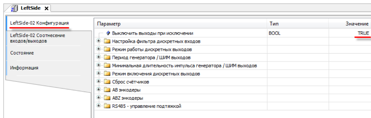
Рисунок 7.33 – Режим обработки выходов при остановке приложения
