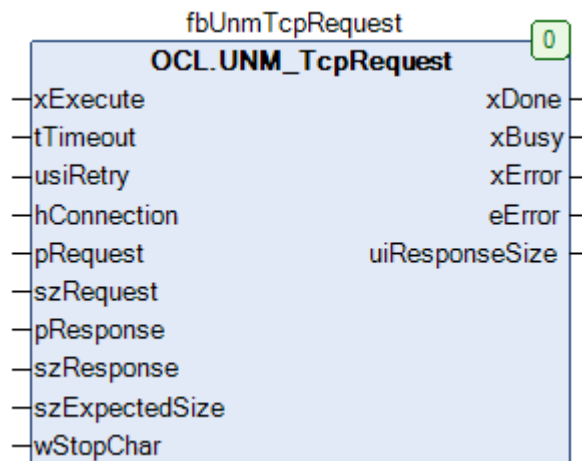
Рисунок 5.1 – Внешний вид ФБ UNM_TcpRequest на языке CFC
