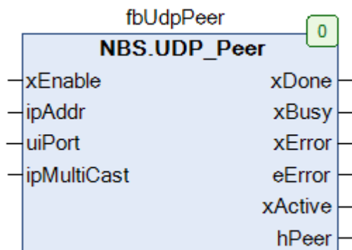
Рисунок 3.2 – Внешний вид ФБ NBS.UDP_Peer на языке CFC
