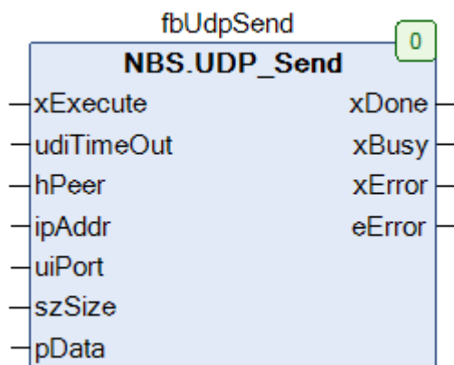
Рисунок 3.4 – Внешний вид ФБ NBS.UDP_Send на языке CFC
