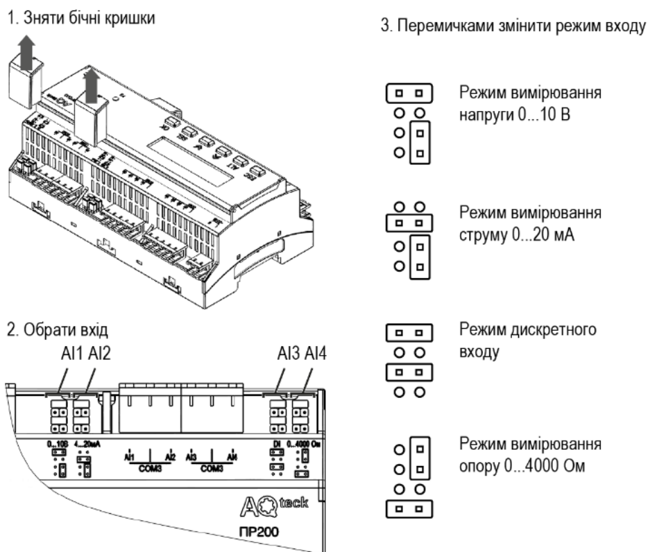
Рисунок 6.3 – Схема розташування перемичок
