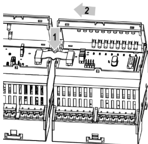
Рисунок 5.13 – Укладання шлейфа в поглиблення
