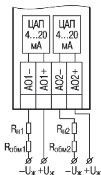
Рисунок 5.10 – Схема підключення навантаження до ВЕ типу «И»
