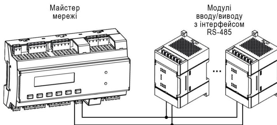
Рисунок 5.16 – Типова схема підключення для ПР200 в режимі Master
