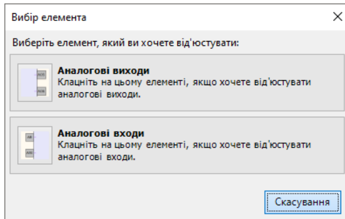
Рисунок 8.6 – Меню юстування
