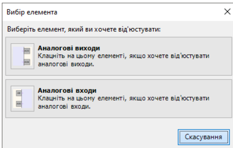
Рисунок 8.11 – Вибір елемента
