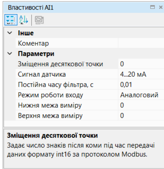
Рисунок 6.2 – Меню параметрів
