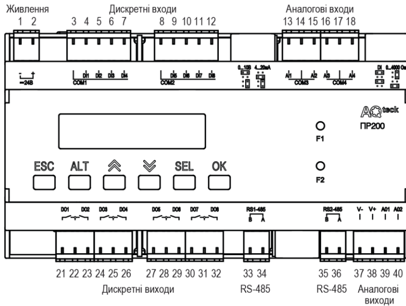
Рисунок А.6 – Розташування контактів ПР200-24.4.2.0
