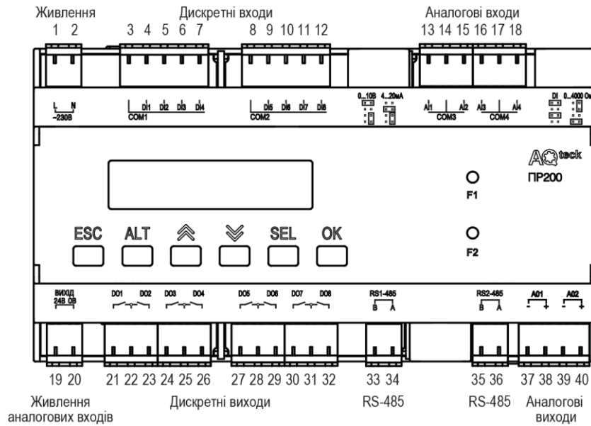
Рисунок А.1 – Розташування контактів ПР200-230.2.2.0
