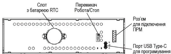
Рисунок 9 – Елементи під лицьовою панеллю
