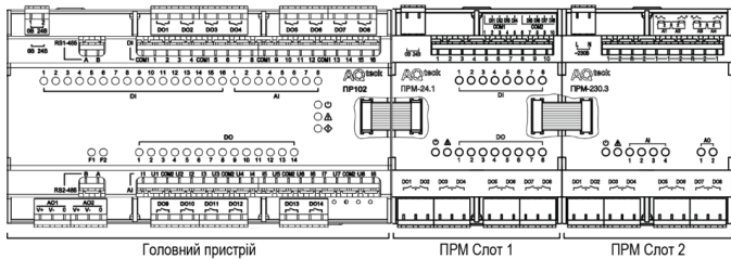
Рисунок 7 – Розташування модулів розширення на шині
