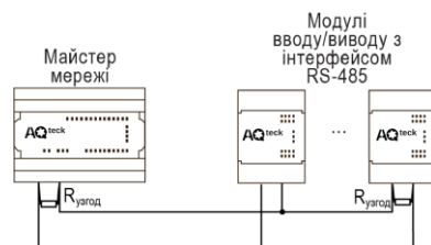
Рисунок 6 – Типова схема підключення у режимі Master
