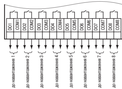
Рисунок 4 – Схема підключення навантажень до ВЕ типу «Р»
