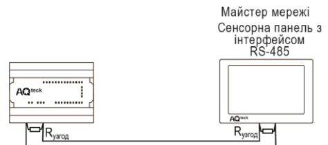
Рисунок 5 – Типова схема підключення у режимі Slave
