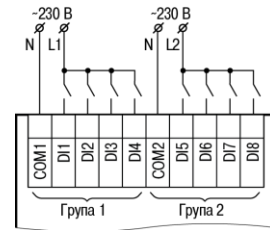
Рисунок 3 – Схема підключення до дискретних входів датчиків типу «сухий контакт» для сигналів 230 В
