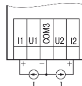
Рисунок 5 – Підключення датчиків з виходом у вигляді струму
