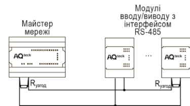
Рисунок 13 – Типова схема підключення у режимі Master
