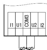
Рисунок 3 – Підключення TO до AI
