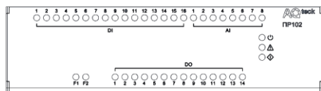
Рисунок 15 – Лицьова панель пристрою
