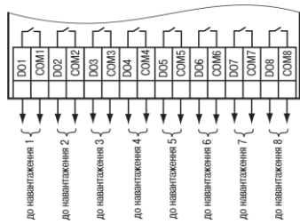
Рисунок 9 – Схема підключення навантажень до ВЕ типу «Р»
