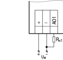
Рисунок 11 – Схема підключення навантажень до ВЕ сигналів «0...10 В»
