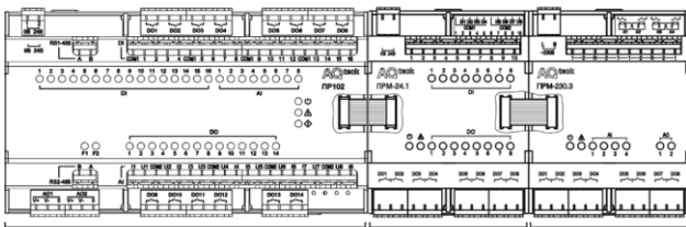
Рисунок 14 – Розташування модулів розширення на шині
