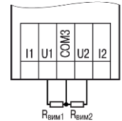
Рисунок 4 – Підключення резистивних датчиків
