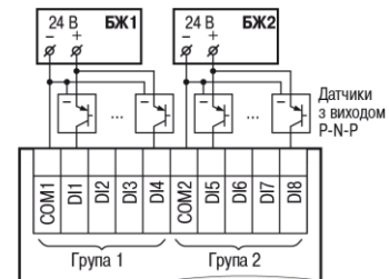
Рисунок 7 – Схема підключення до дискретних входів, що працюють у дискретному режимі, трипровідних дискретних датчиків, які мають вихідний транзистор р-п-р-типу з відкритим колектором для сигналів 24 В
