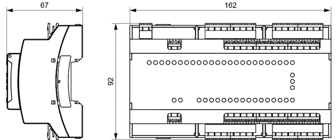
Рисунок 2 – Габаритні розміри пристрою
