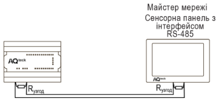
Рисунок 12 – Типова схема підключення у режимі Slave
