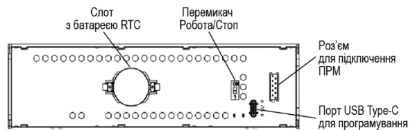
Рисунок 16 – Елементи під лицьовою панеллю
