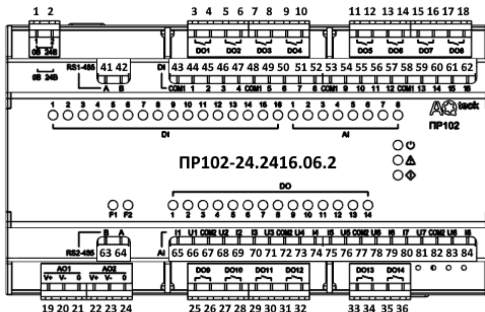
Рисунок А.4 – Розташування контактів для ПР102-24.2416.06.2
