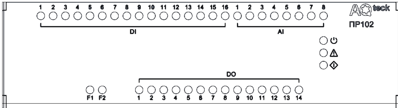
Рисунок 7.1 – Лицьова панель пристрою
