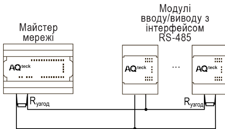
Рисунок 6.17 – Типова схема підключення у режимі Master
