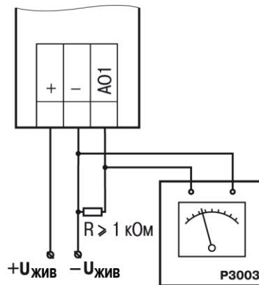
Рисунок Б.8 – Схема підключення навантаження до ВЕ для юстування сигналів типу «0...10 В»
