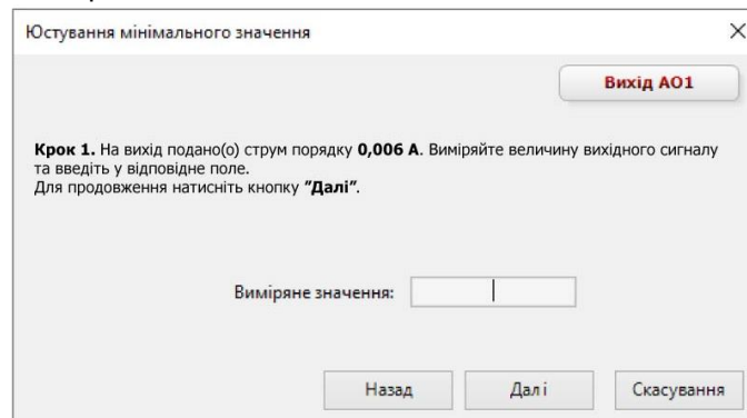
Рисунок Б.7 – Калібрування мінімального значення
