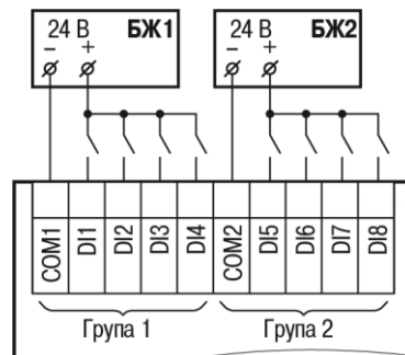
Рисунок 6.2 – Підключення до дискретних входів датчиків типу «сухий контакт» для сигналів 24 В
