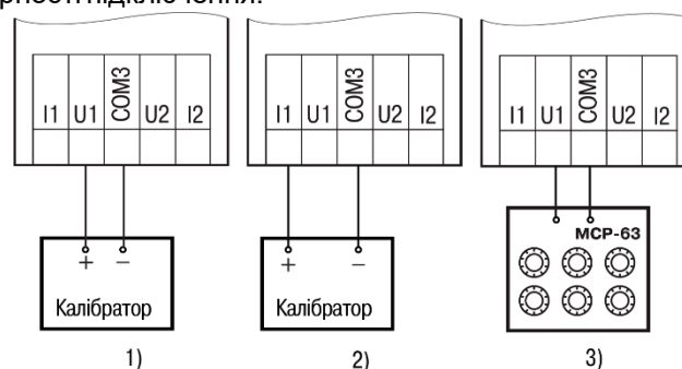
Рисунок Б.1 – Підключення джерела еталонного сигналу
