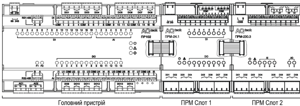
Рисунок 6.15 – Розташування модулів розширення на шині
