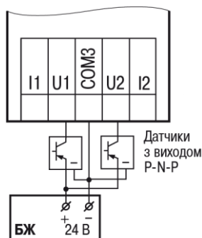
Рисунок 6.5 – Схема підключення до універсальних входів, що працюють у дискретному режимі, трипровідних дискретних датчиків, які мають вихідний транзистор р-п-р-типу з відкритим колектором
