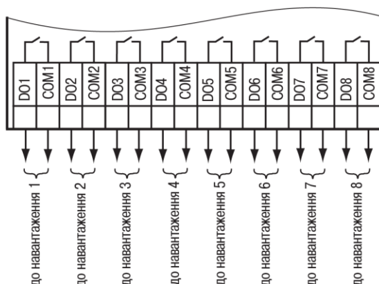
Рисунок 6.11 – Схема підключення навантаження до ВЕ типу «Р»
