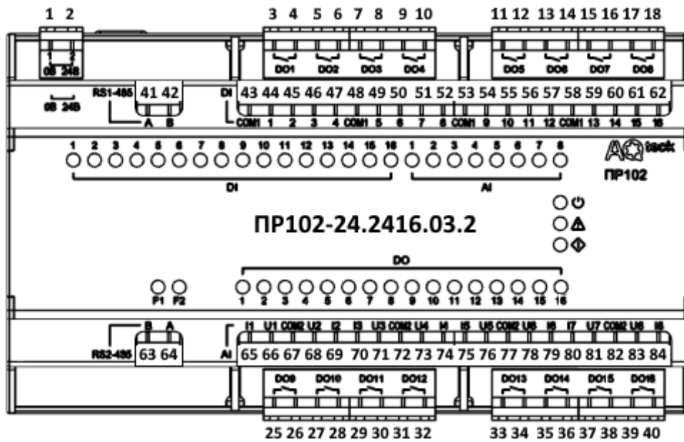
Рисунок А.2 – Розташування контактів для PR102-24.2416.03.2
