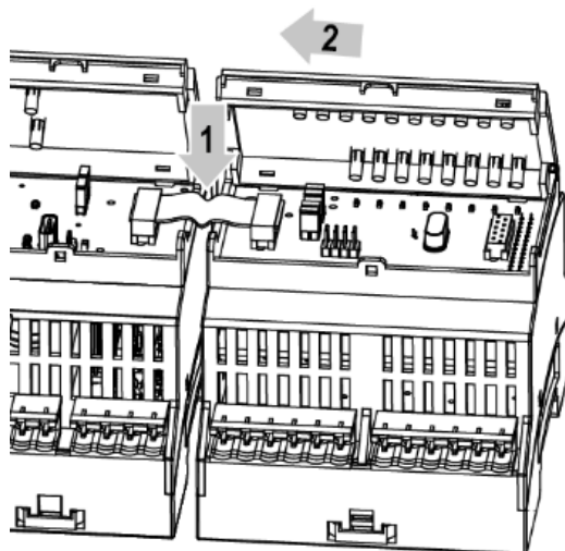
Рисунок 6.14 – Укладання шлейфа у поглиблення
