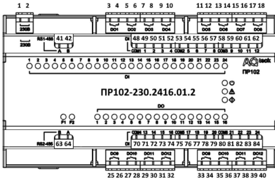
Рисунок А.1 – Розташування контактів для ПР102-230.2416.01.2
