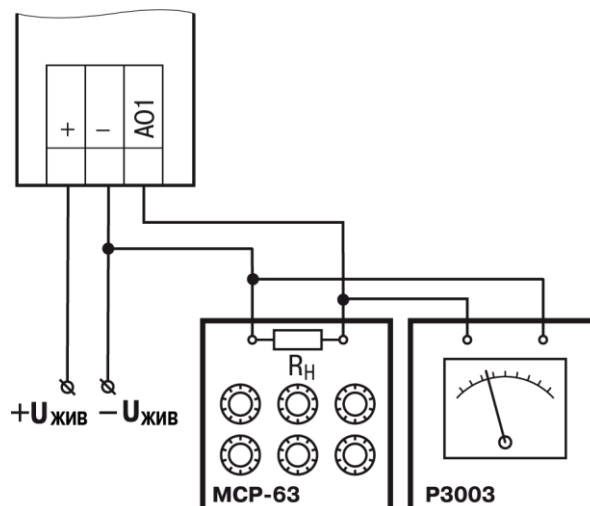
Рисунок Б.4 – Схема підключення до ВЕ для юстування сигналів типу «4...20 мА» ( R_n < 300 \text{ Ом} )
