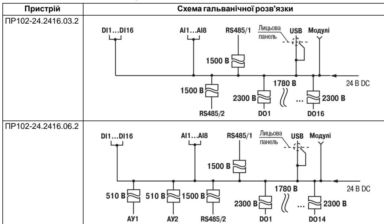
Таблиця 6.2 – Схеми гальванічної розв'язки ПР102-24.2416.х.2
