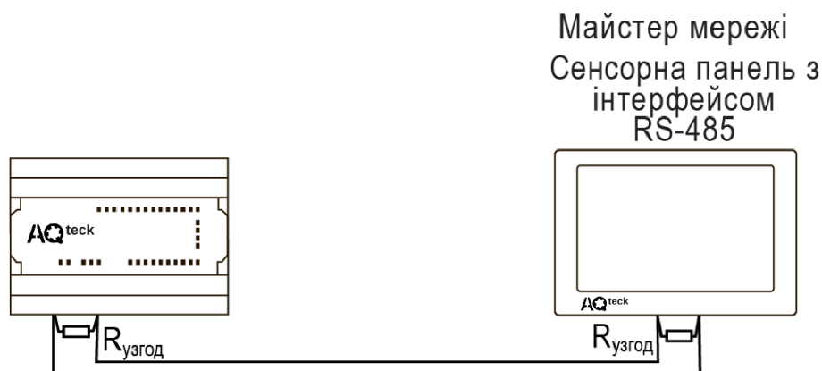
Рисунок 6.16 – Типова схема підключення у режимі Slave
