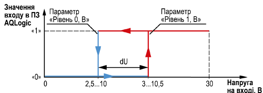
Рисунок 4.3 – Робота універсального входу у дискретному режимі
