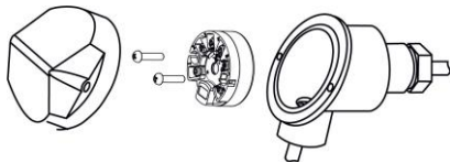
Рисунок 6.2 – Монтаж пристрою
