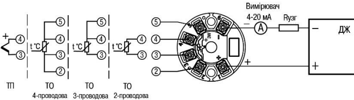
Рисунок 6.3 – Підключення пристрою
