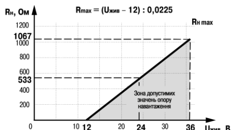
Рисунок 2.1 – Графік для вибору допустимих значень опору навантаження
