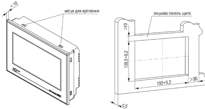
Рисунок 3 – Установчі розміри СП307
