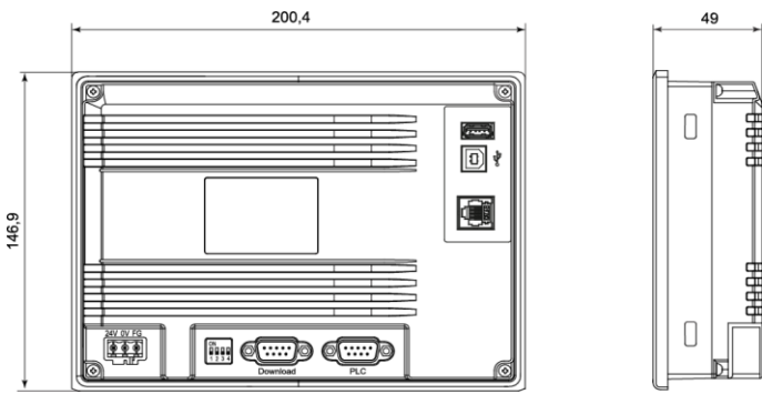
Рисунок 2 – Габаритні розміри СП307
