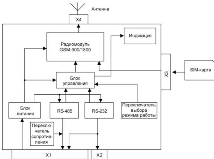
Рисунок 3.1 – Функциональная схема
